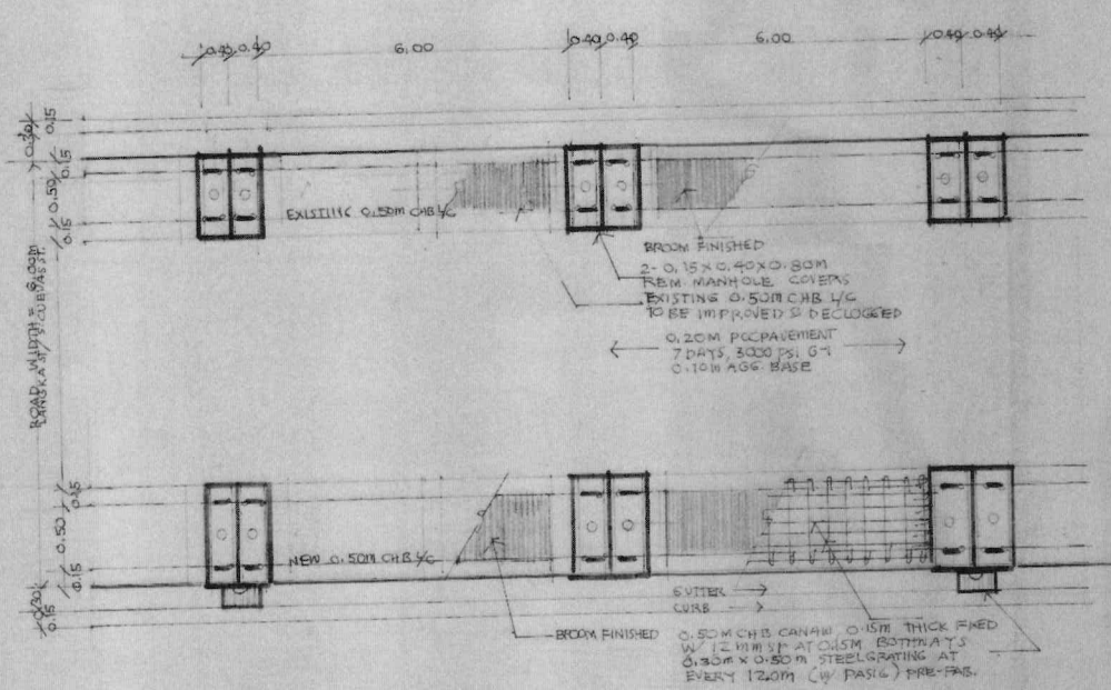
PLAN OF CHB 1/2 S. CUEVAS ST. / LANGKA ST.
